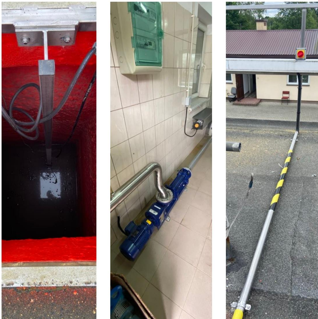
Rysunek 20 Wykonana modernizacja oczyszczalni ścieków w Wilczej Woli
